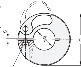
Voreinstellschraube
